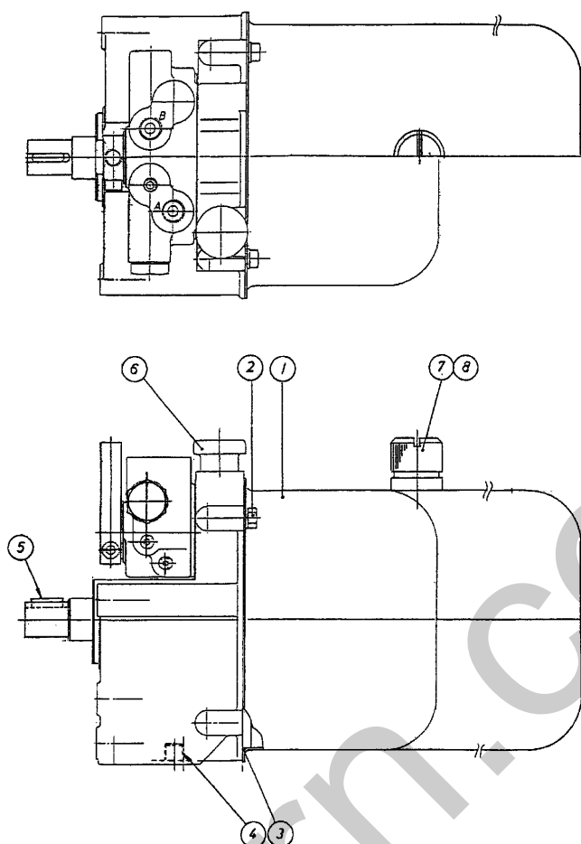
FIG 20 パッケージ HYDRAULIC PUMP ~NO.6140016
