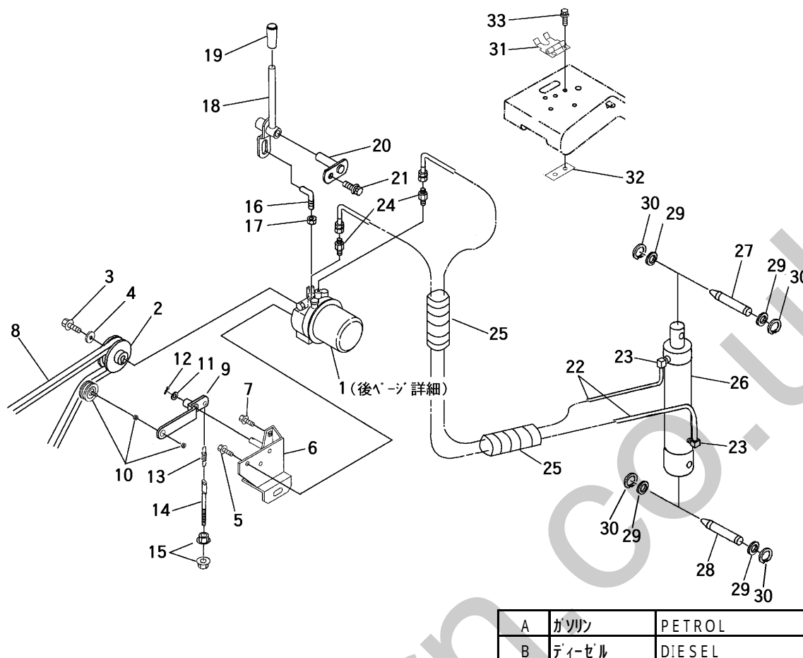
FIG 16 ユアツソウチ HYDRAULIC LINE
