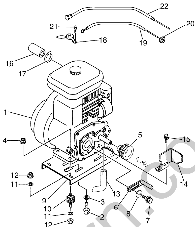
FIG 1 エンジン&エンジンコントロール(クボタ ガソリン) ENGINE & ENGINE CONTROL (KUBOTA PETROL)
