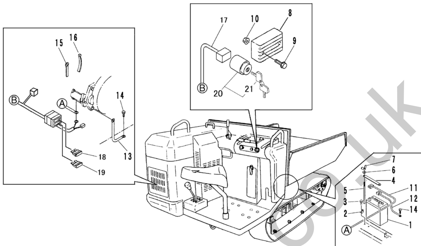
FIG 3 デンソウ ( ソノ1 ) ELECTRIC EQUIPMENT ( PART-1)
