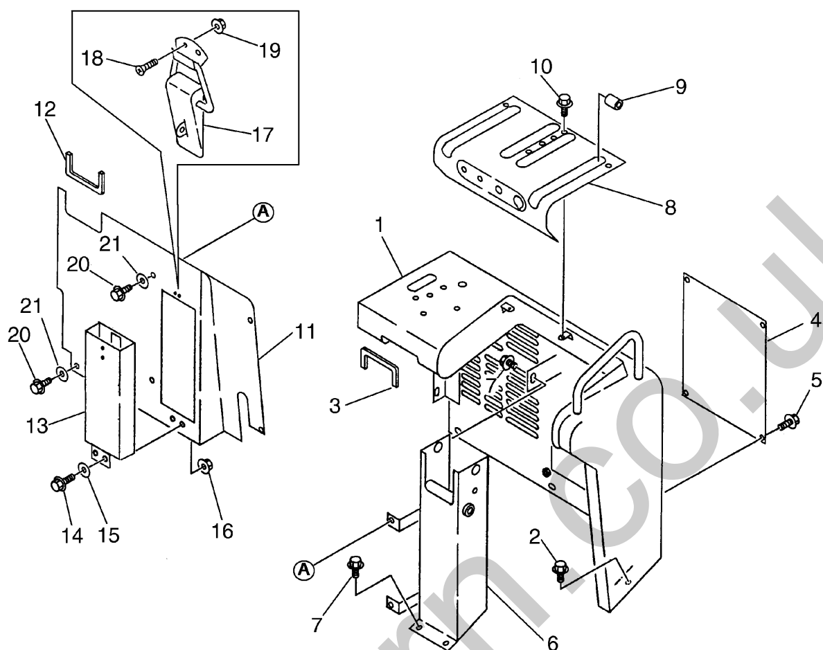
FIG 6 ウンテンセキカバー CAB COVER
