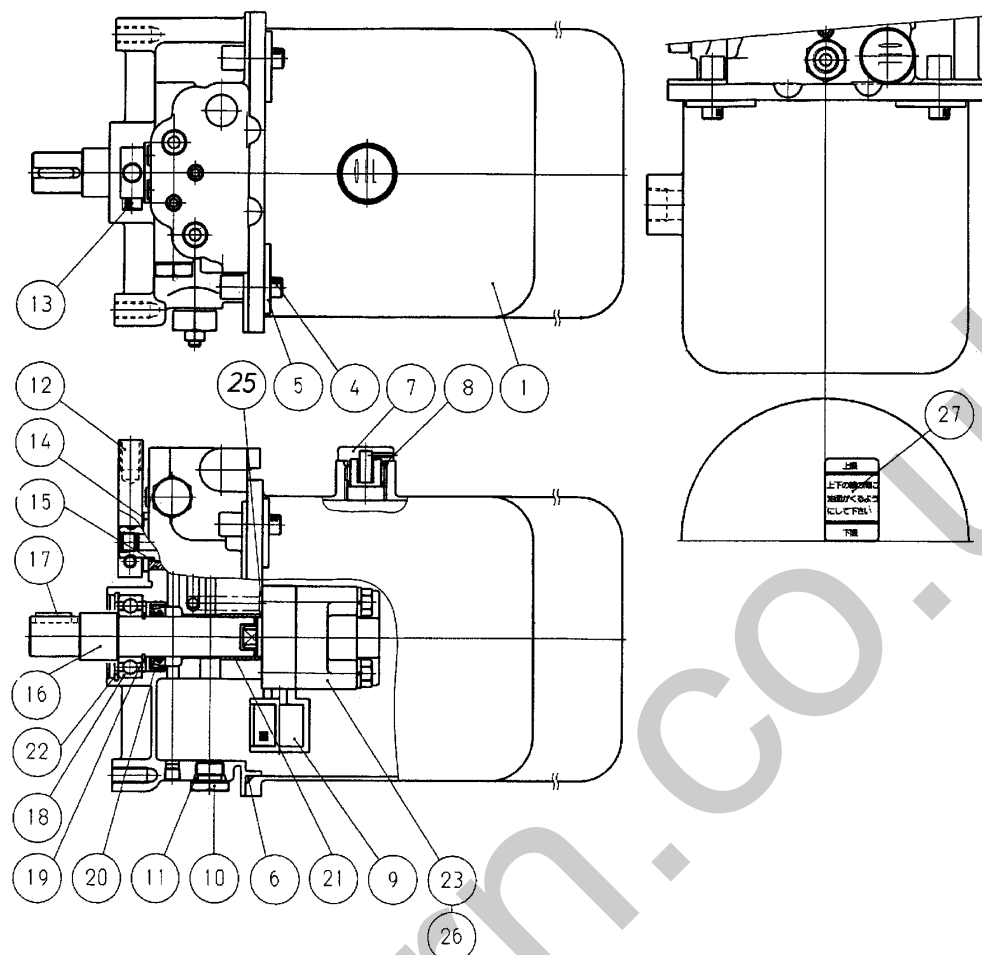
FIG 19 パッケージ HYDRAULIC PUMP NO.6140017~
