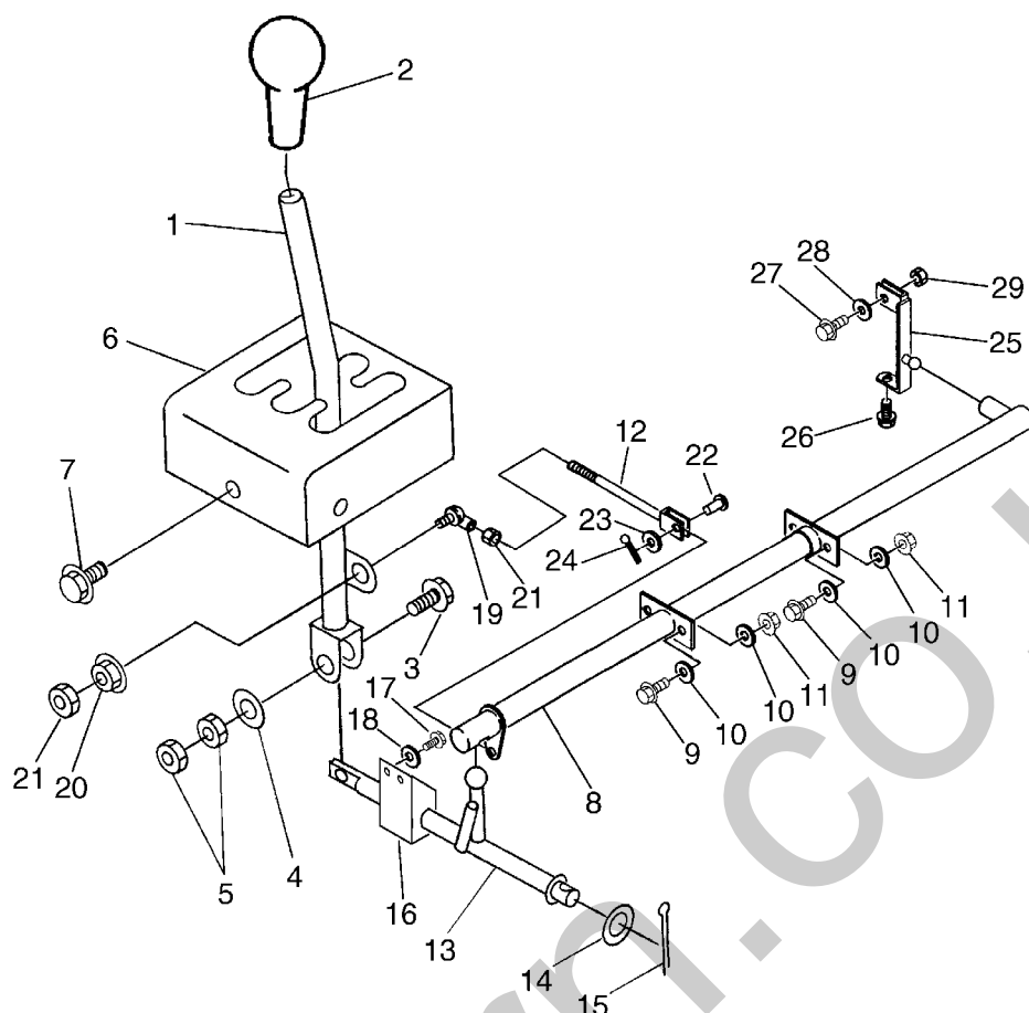
FIG 13 チェンジ GEAR SHIFT LEVER
