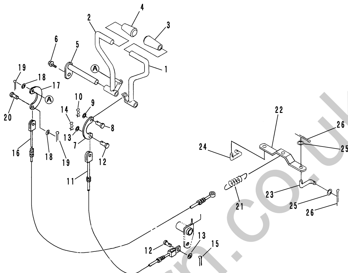
FIG 12 ブレーキ & クラッチレバー BRAKE & CLUTCH LEVER
