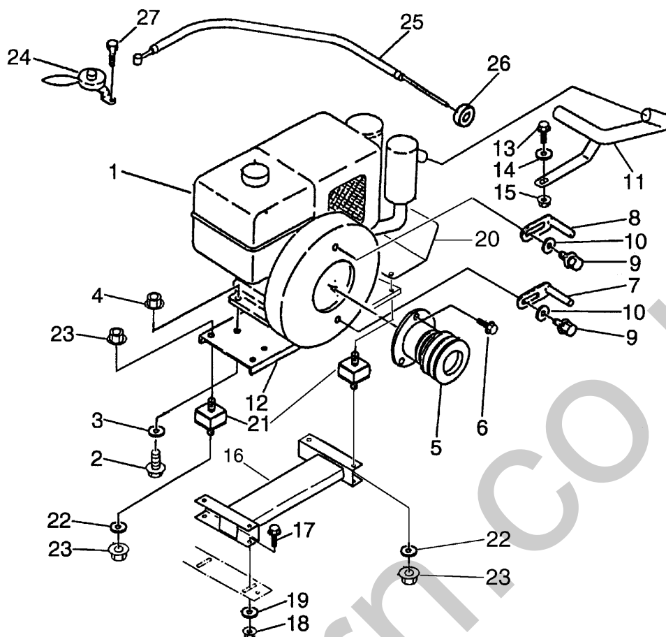
FIG 2 エンジン&エンジンコントロール(クボタ ディーゼル) ENGINE & ENGINE CONTROL (KUBOTA DIESEL)
