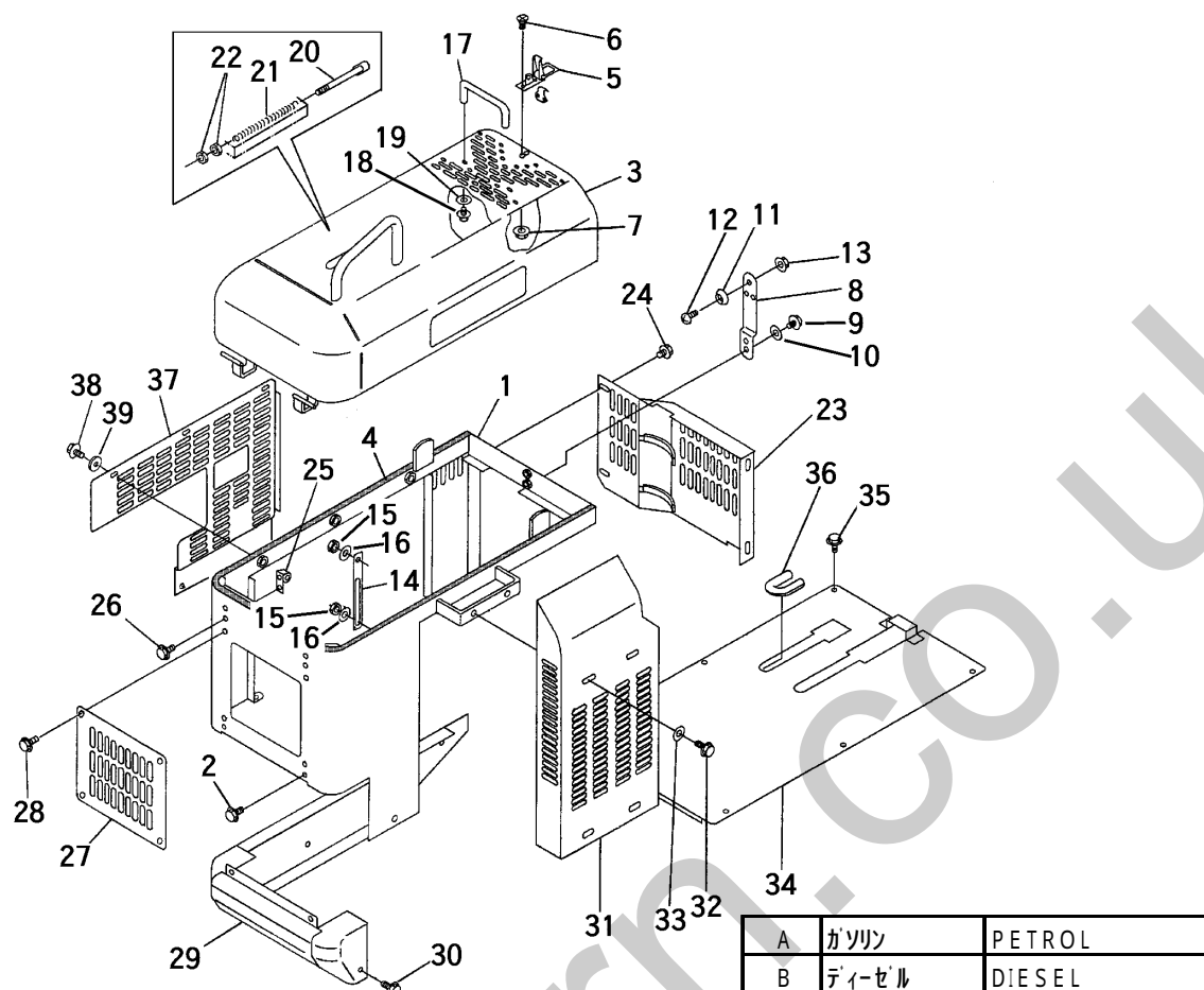
FIG 7 エンジンカバー ENGINE COVER
