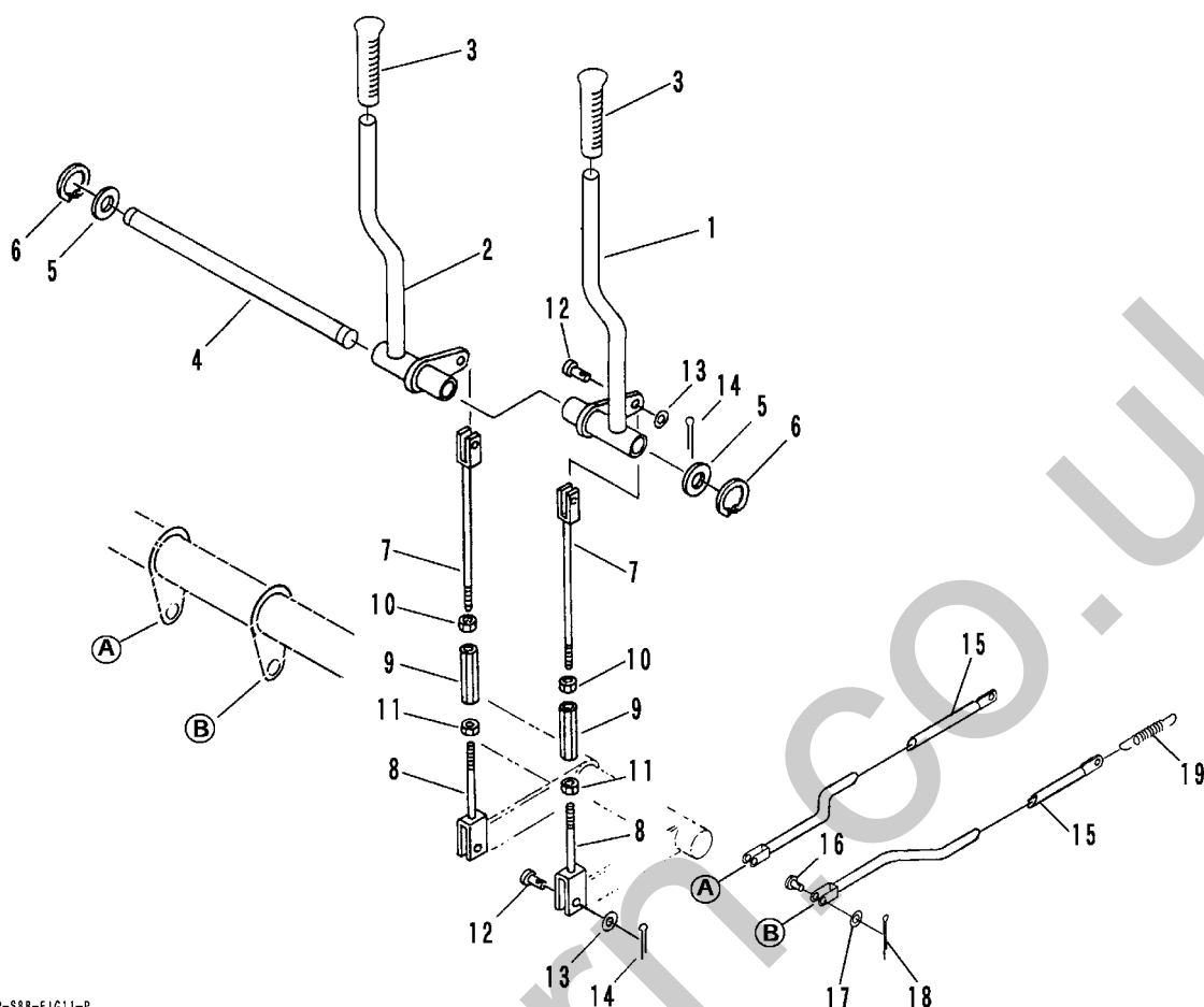
FIG 11 サイドクラッチレバー SIDE CLUTCH LEVER
